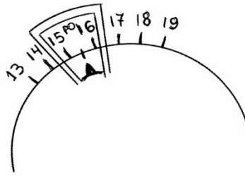
Fig. 17. Trazado de índice en el sector graduado
