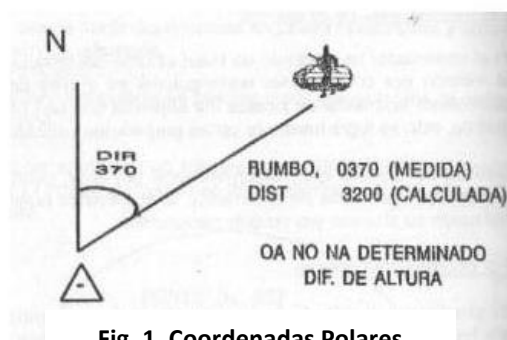
Fig. 1. Coordenadas Polares
