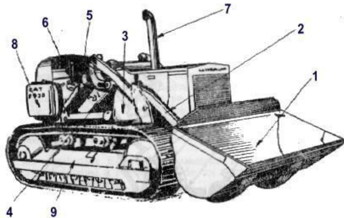
Figura 2. Nomenclatura del cargador frontal a orugas 977 H CAT.
