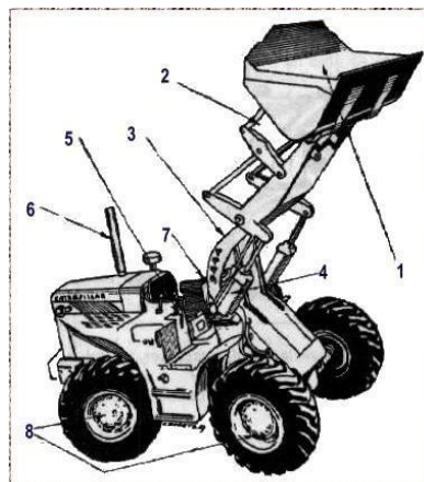
Figura 1. Nomenclatura del cargador frontal a ruedas 944 A CAT.
